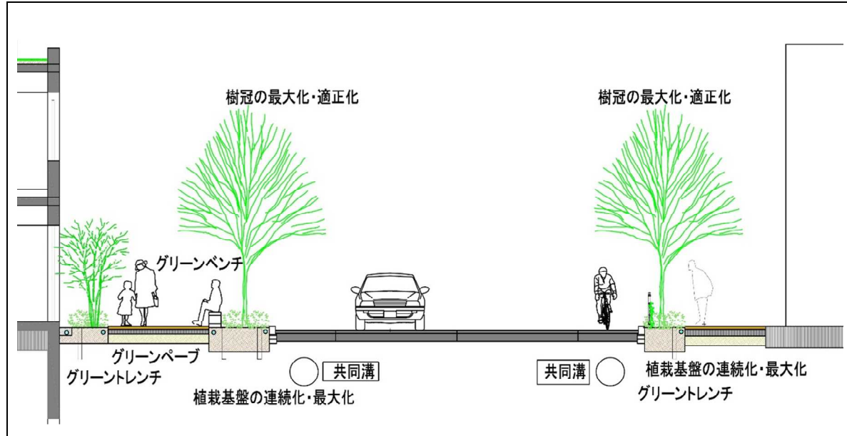
・エコグリーンロードの断面模式図
